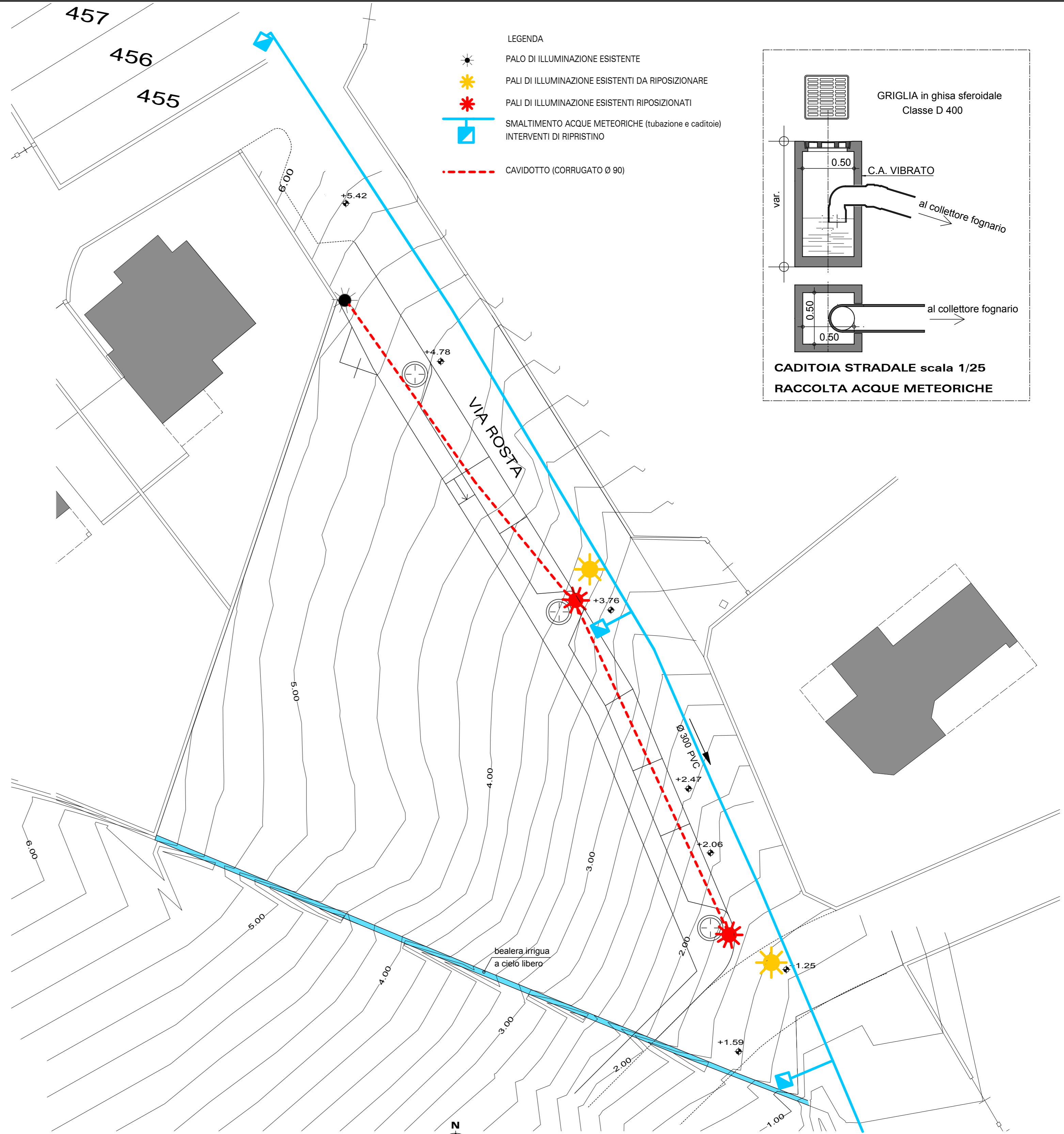
PLANIMETRIA - PROGETTO NUOVE OPERE DI URBANIZZAZIONE scala 1/200
